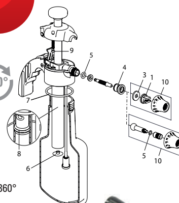
Buse à mousse G3/8"
