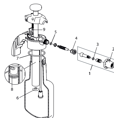
Set d'anneaux pour Super Spray-Matic 1.0 N 12164201
